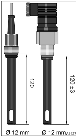
Fig. 1: Dimensions
